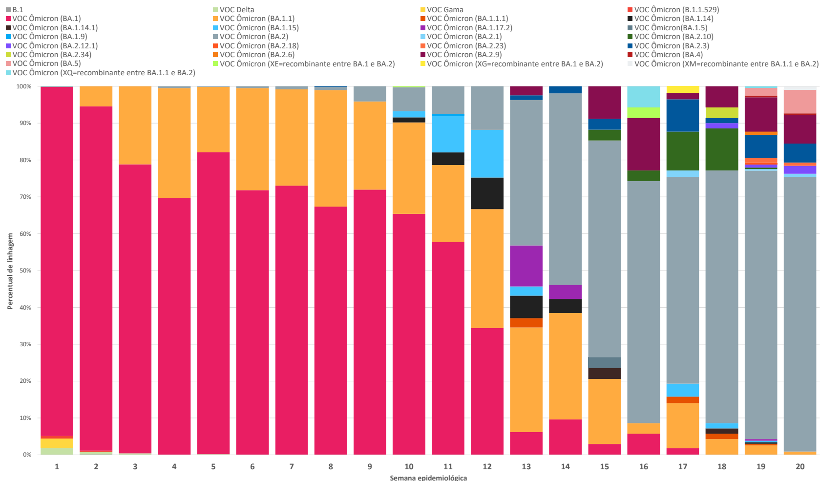
GRÁFICO 3. Variantes do SARS-CoV-2 por semana epidemiológica no estado de São Paulo – Instituto Butantan, 2022
